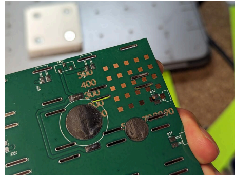
(d) soldermask-array
